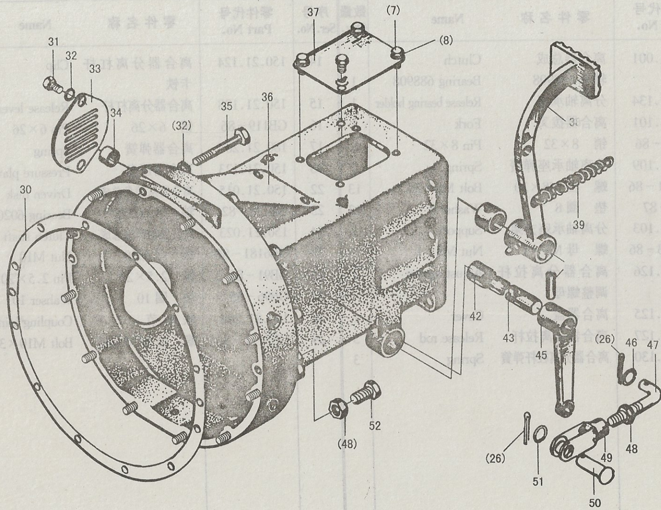
图 3. 离合器总成 Fig.3 Clutch
