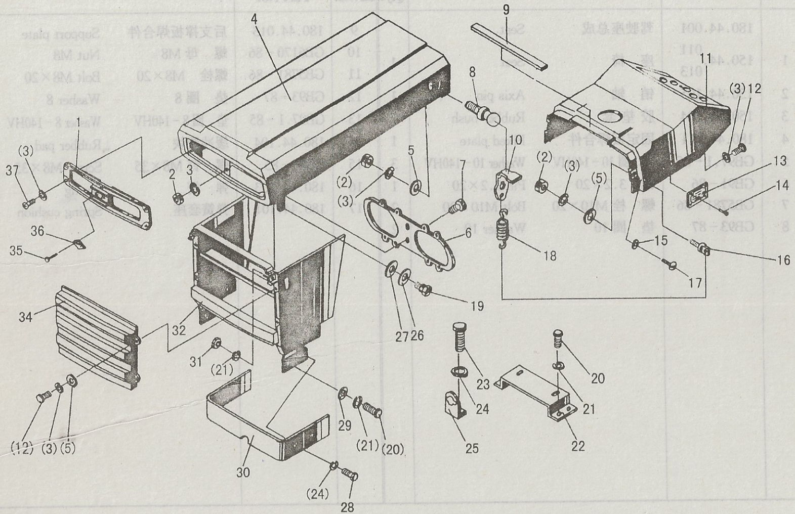
图 13. 机罩、仪表盘总成
