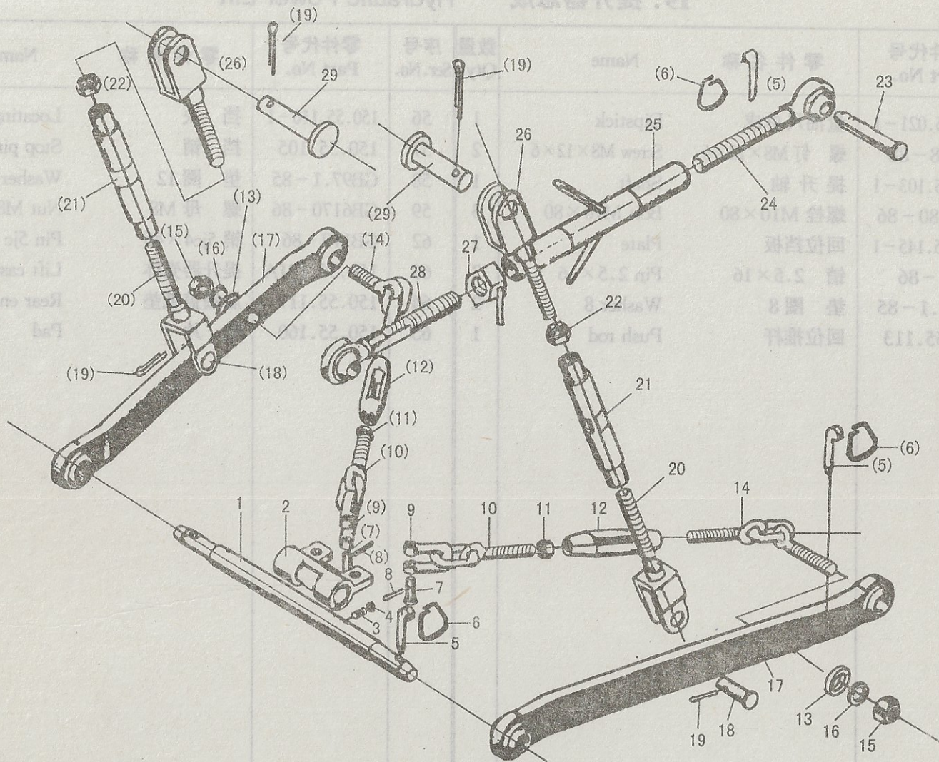
图 20. 悬挂机构总成
