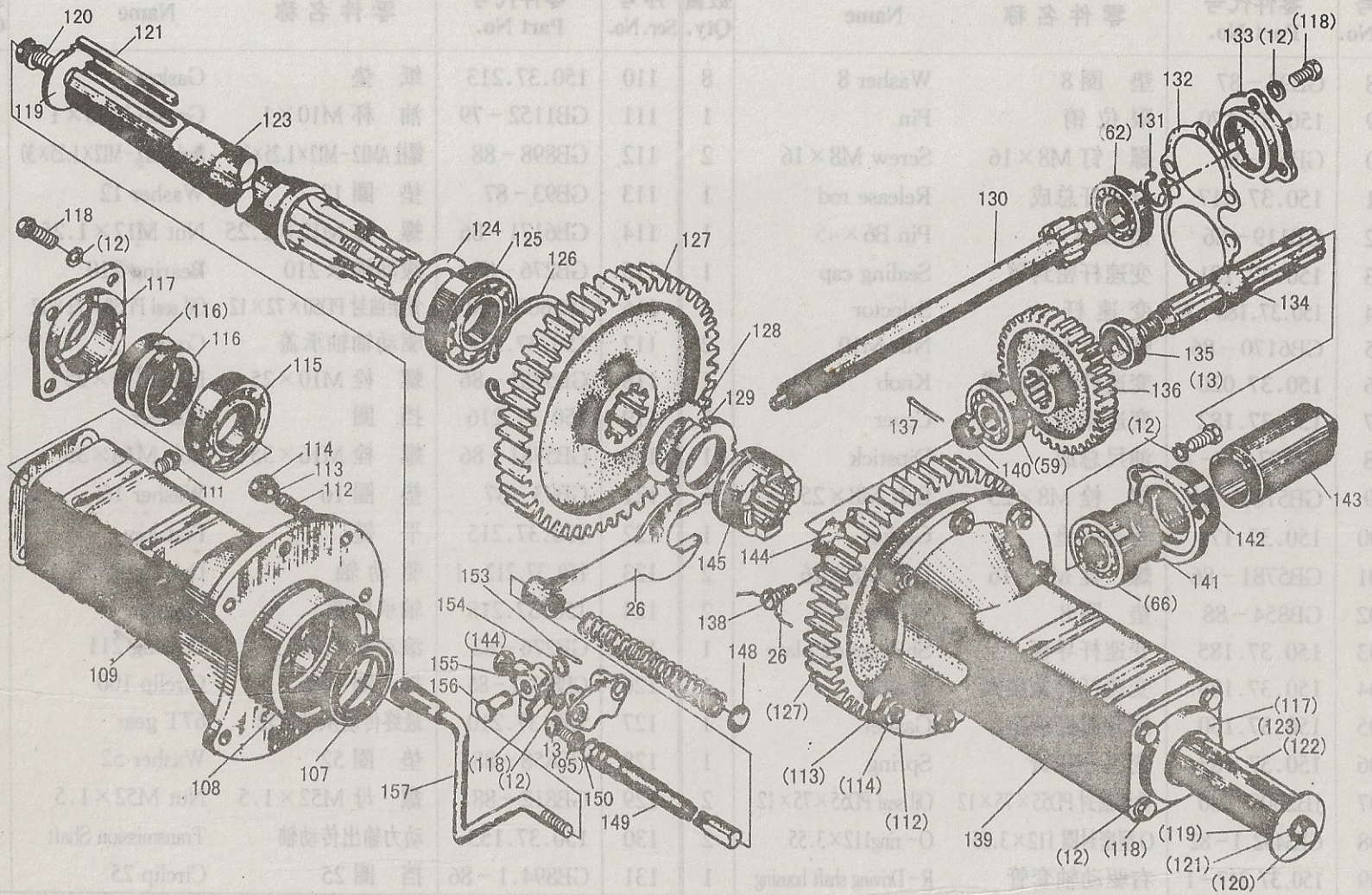
图 9. 传动箱总成
