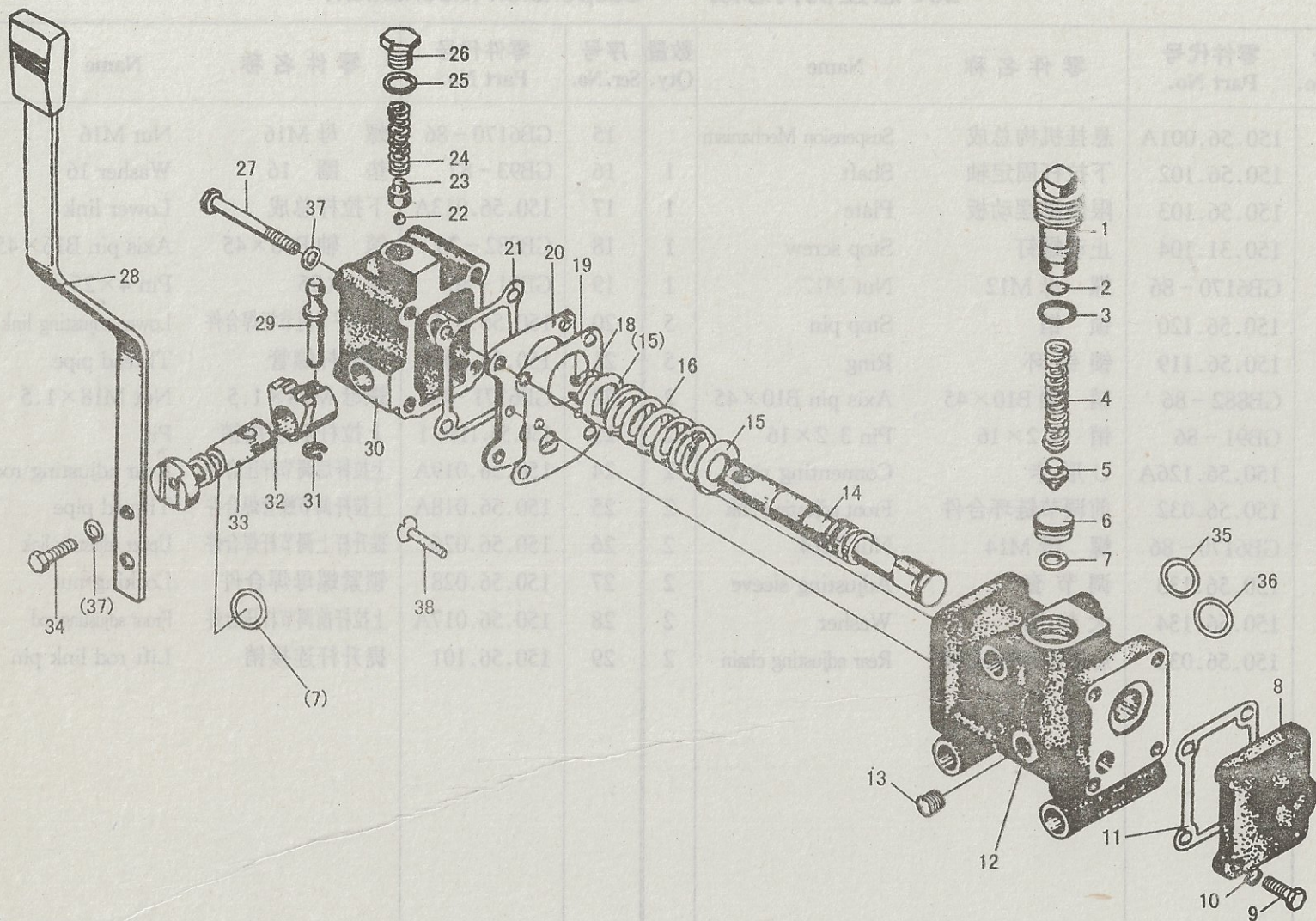
图 21. 分配器总成
