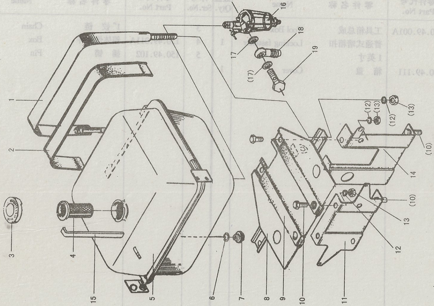
图 17. 燃油箱总成 Fig.17 Fuel Tank
