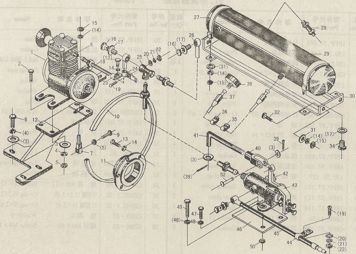
图 22. 180 拖车气制动总成
