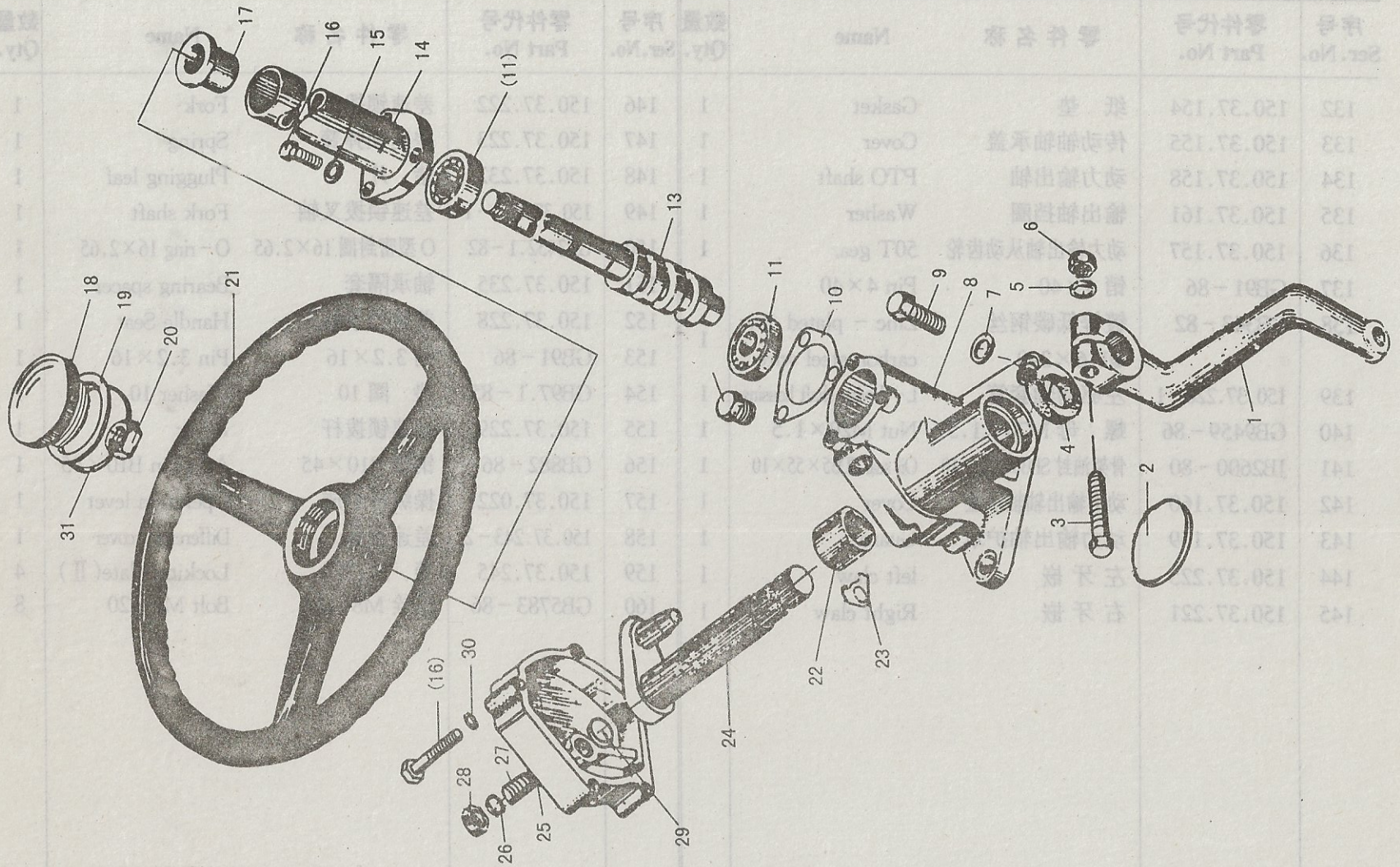
图 10. 转向器总成
